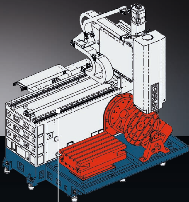
U5-1530 [Наклонно-поворотный стол]
