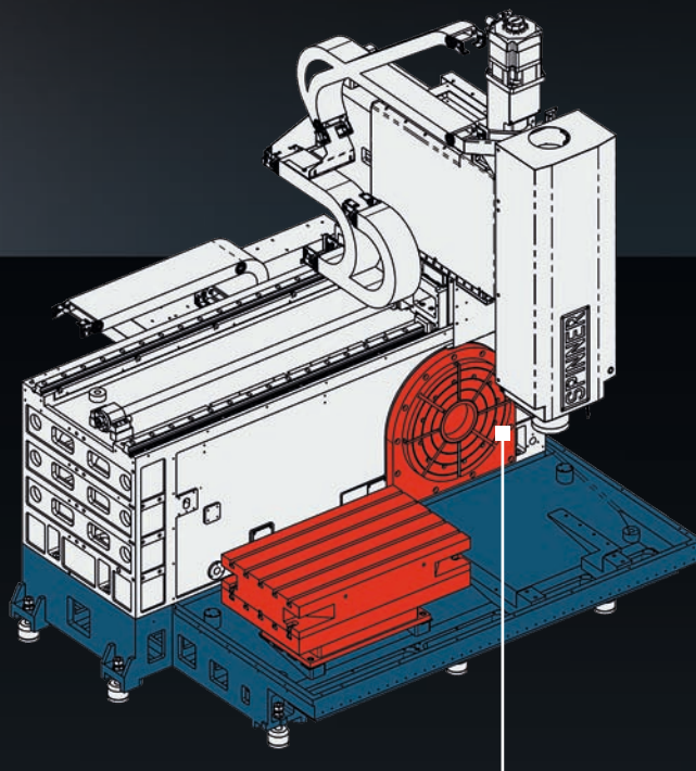
U4-1530 [Поворотный стол]
