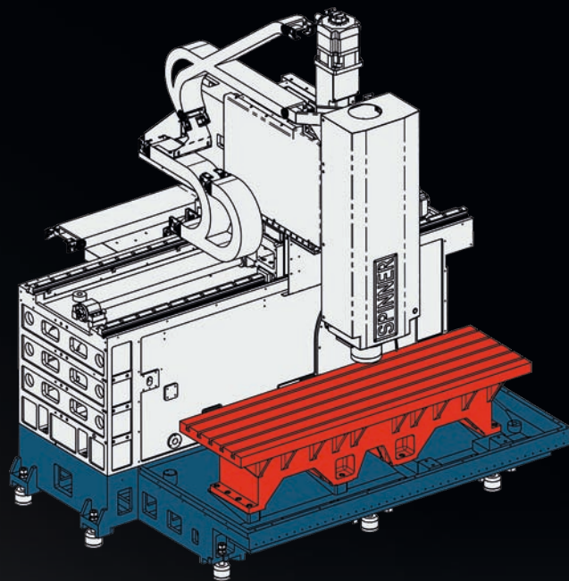
U4-1530 [Поворотный стол]
